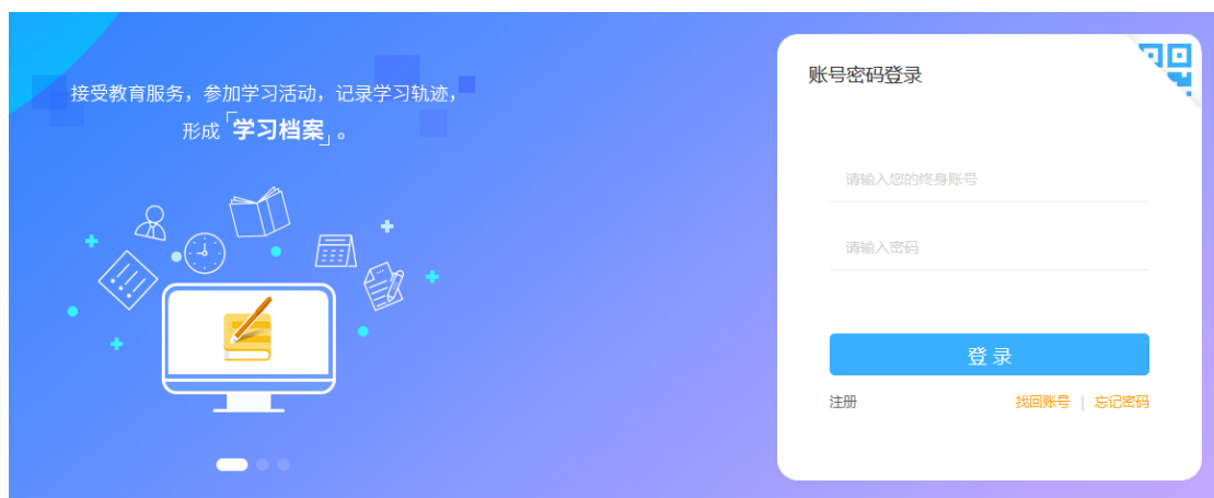
图1-1 登录界面
