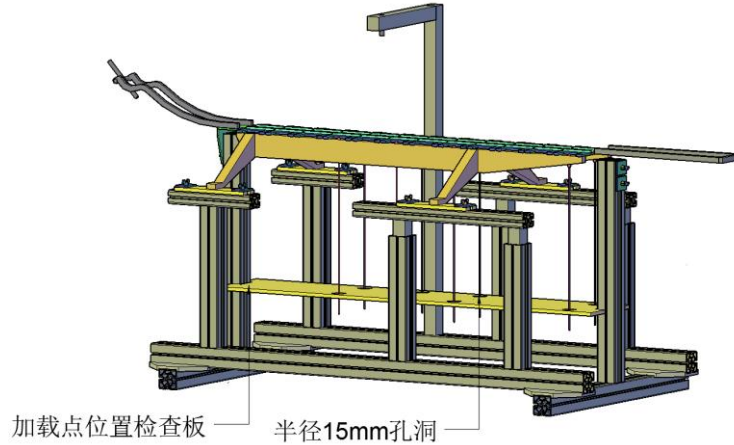
图11 辅助安装装置示意
